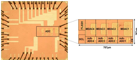
Fig. 21. ADC die photograph.
